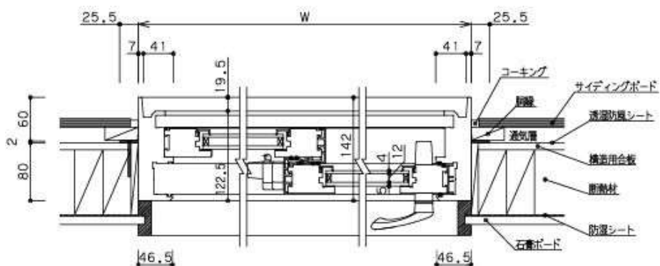
横断面図
