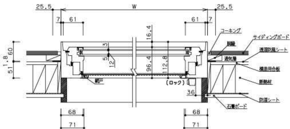
横断面図
