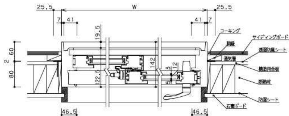
横断面図
