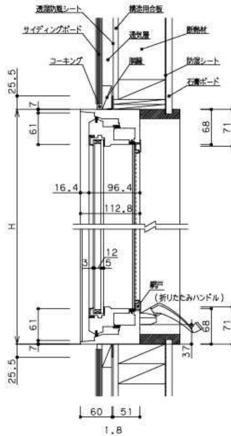
縦断面図
