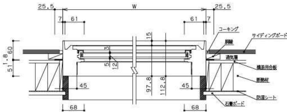
横断面図
