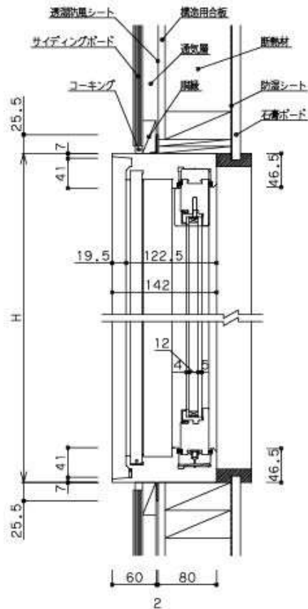
縦断面図 (可動部)
