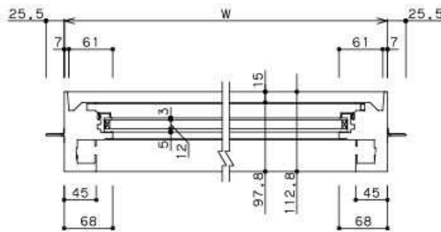
縦断面図
