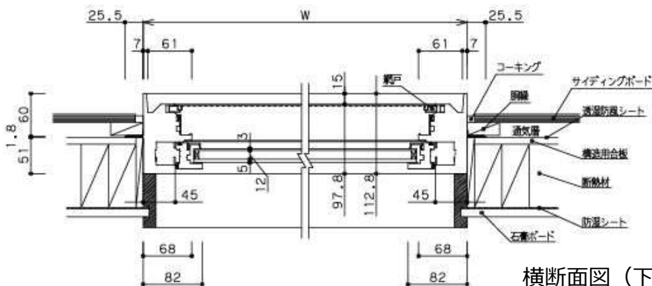
横断面図 (上部: FIX部)
