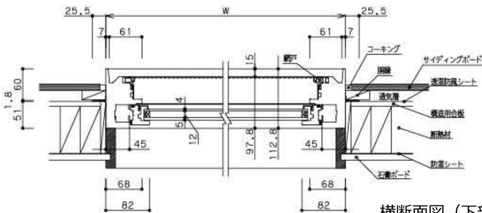
横断面図 (上部: FIX部)
